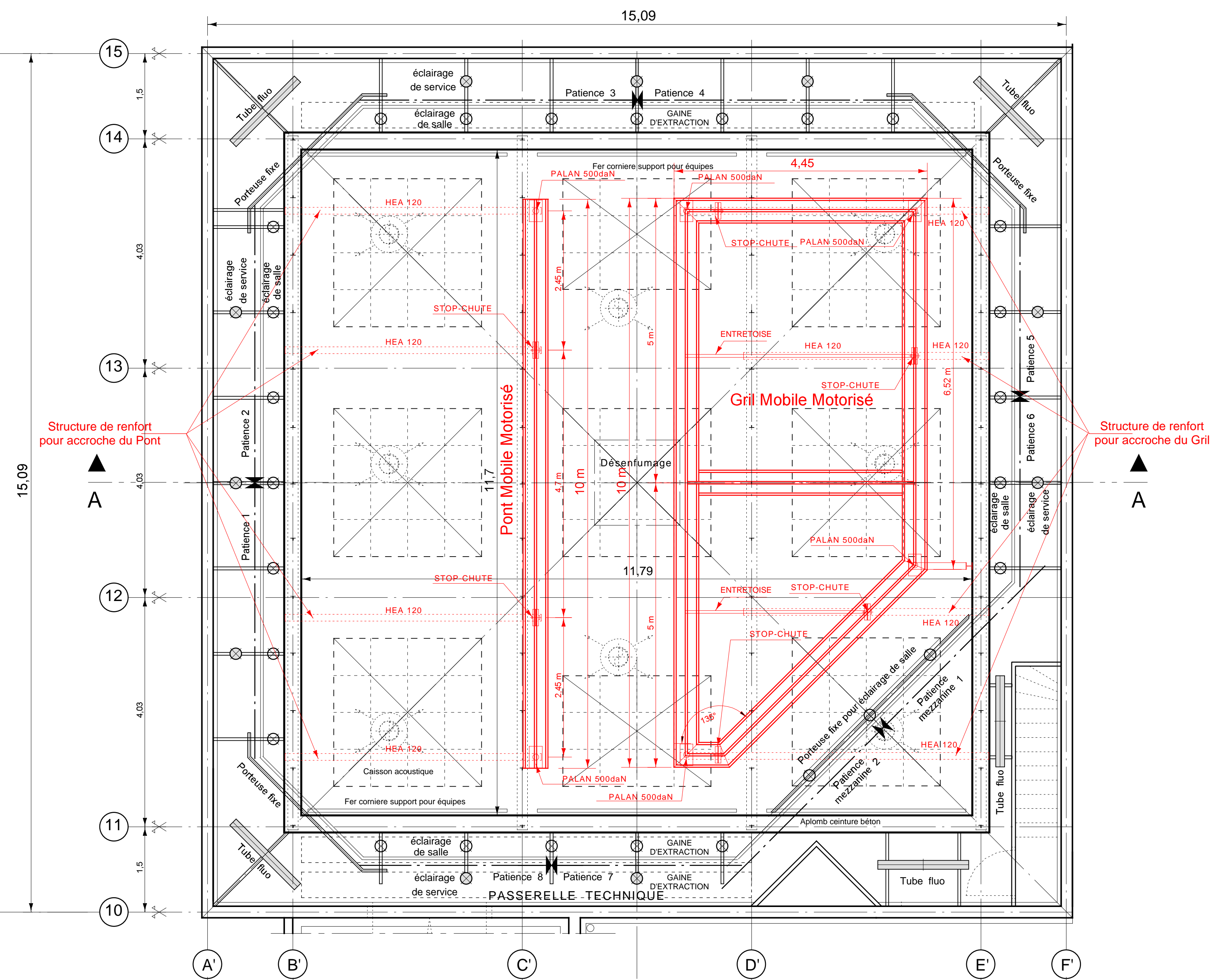
PLAN du FAUX - PLAFOND
