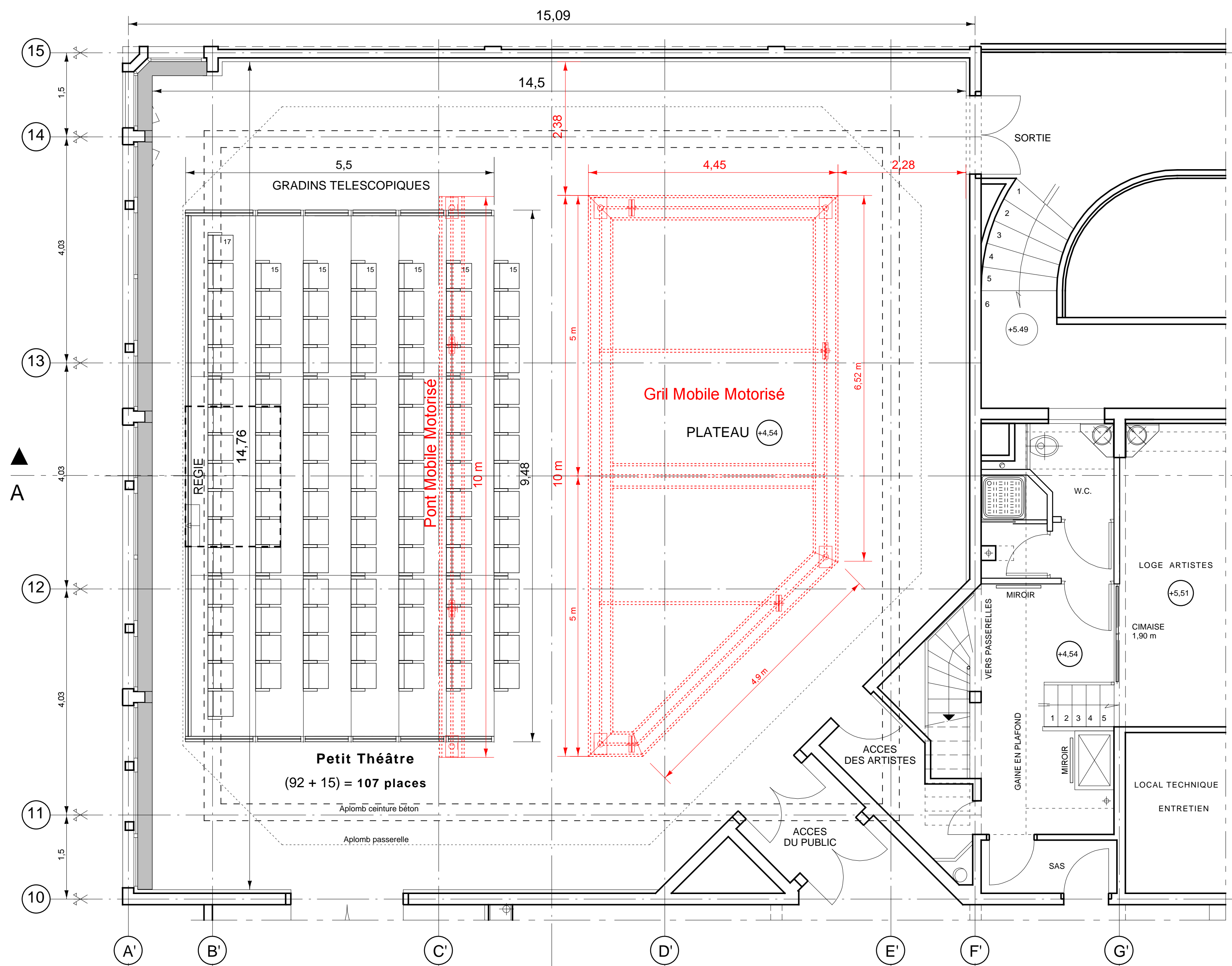
PLAN du PLATEAU
